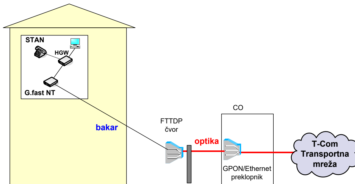
Slika 36a. Način realizacije FTTDP koncepta sa G.fast tehnologijom u pristupnoj mreži
